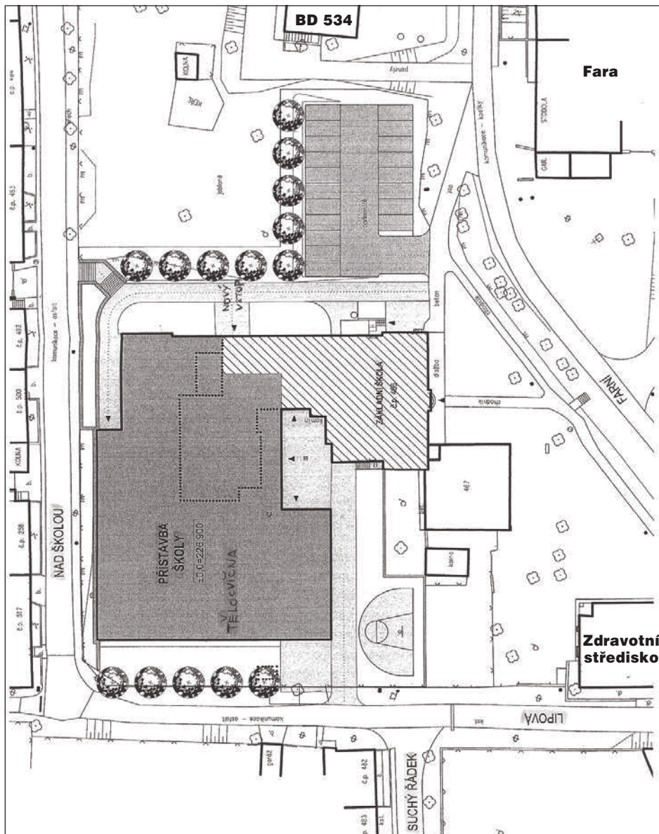
Situace: Stavební úprava a přístavba objektu školy Dambořice
