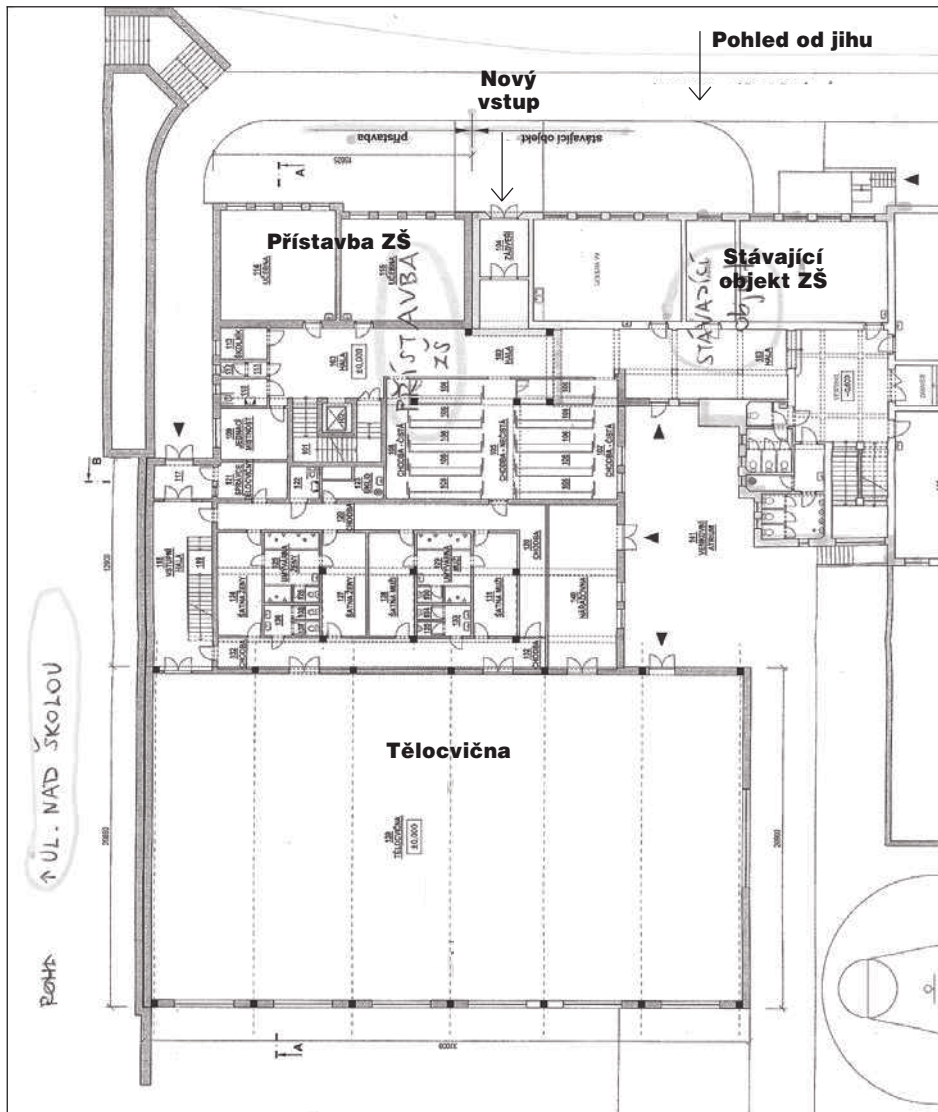
Půdorys tělocvičny a nové části přístavby
